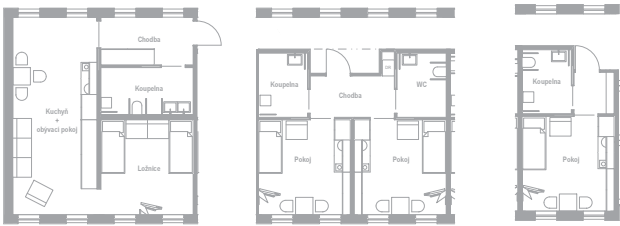
Dvoulůžkový pokoj M 1:100
